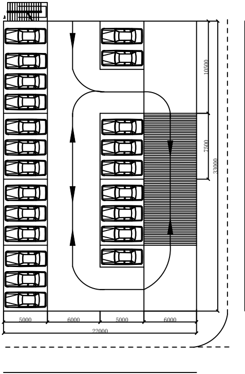
二层平面图：停车数量22个泊位
