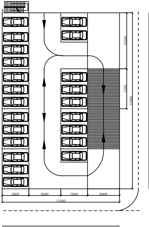
三层平面图：停车数量22个泊位
